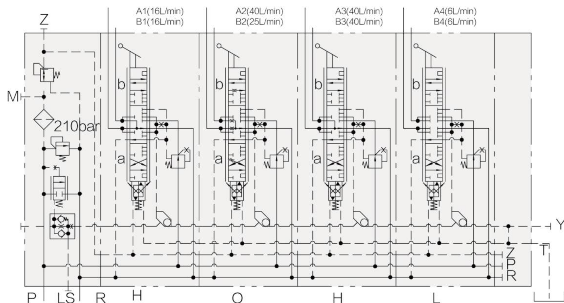
液压原理图
