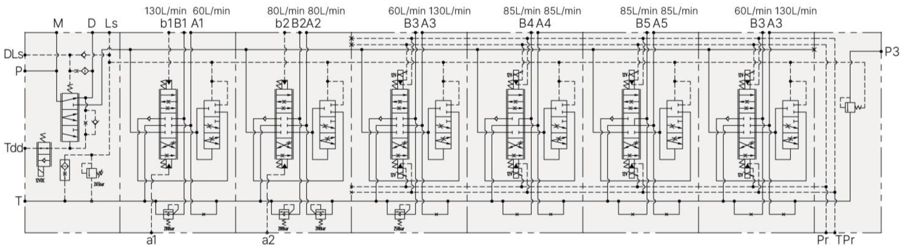
液压原理图
