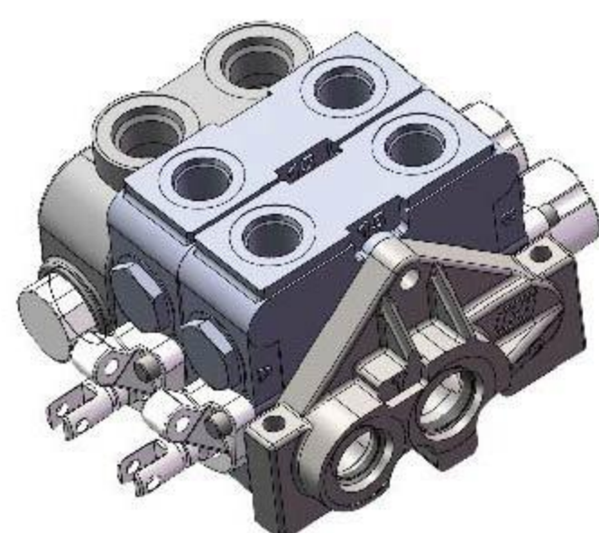
SDV*-25 系列多路换向阀 DIRECTIONAL VALVE
